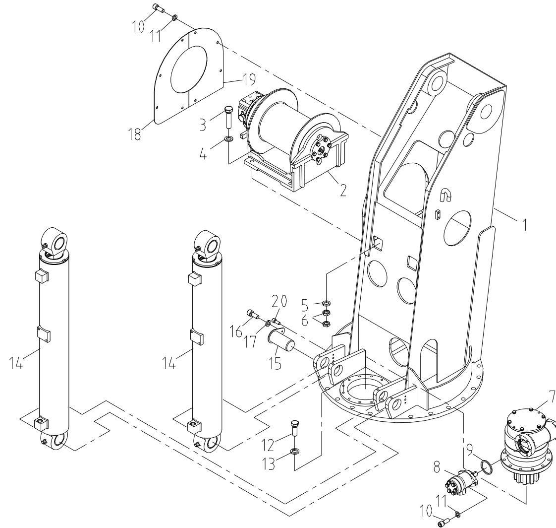
스윙 포스트 조립체 Fig. 2 SCS1024LSuper SWING POST ASS'Y
