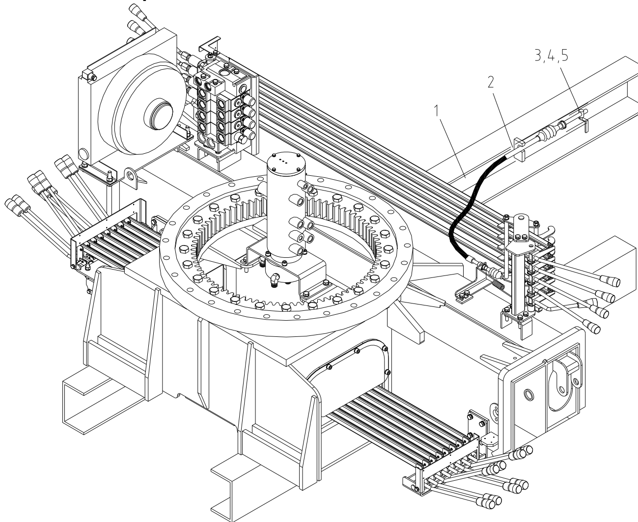
악셀 시스템 파트 Fig. 8-3 SCS1024LSuper ACC'L SYSTEM PART
