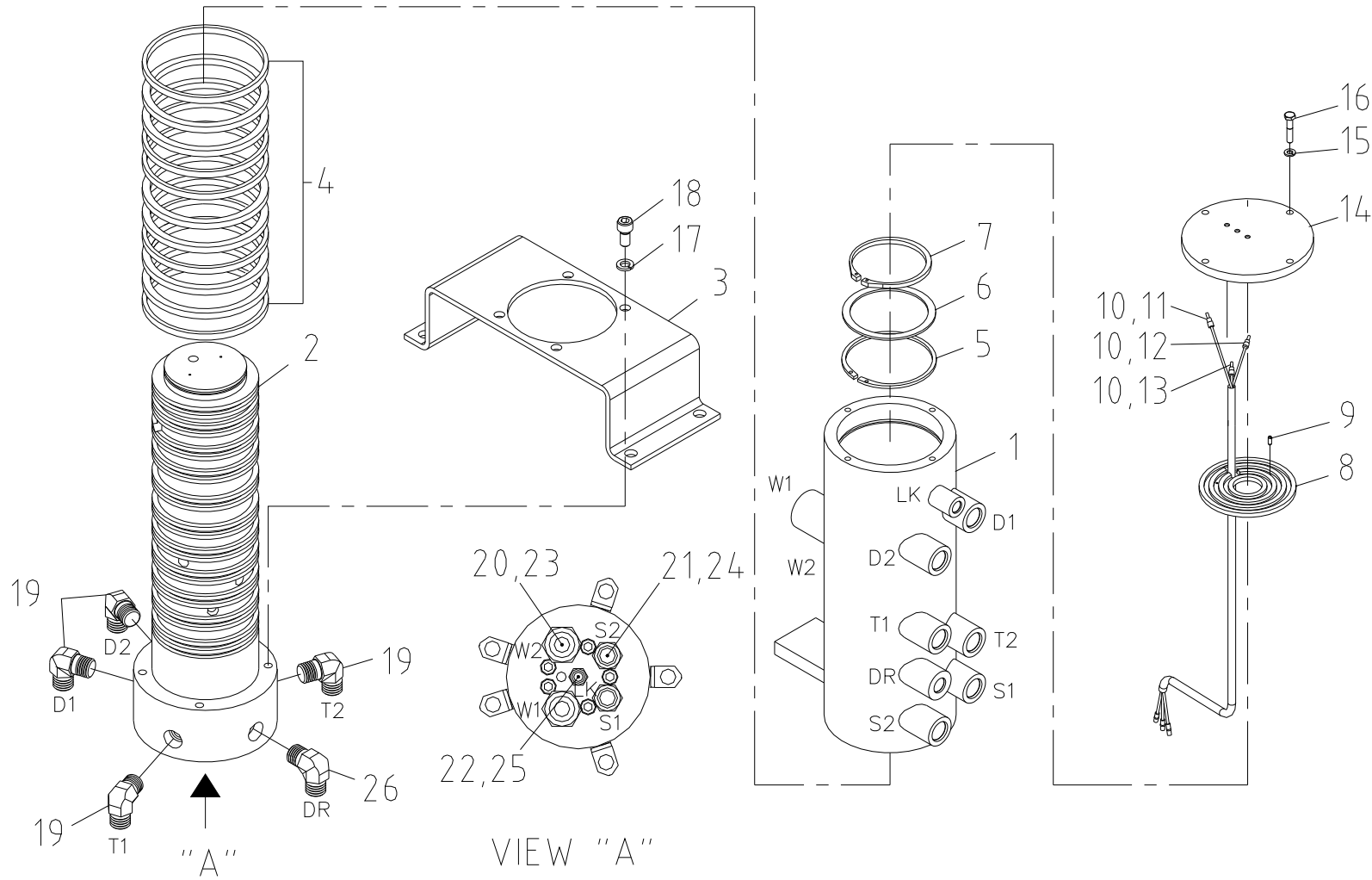
로타리 조인트 조립체 Fig. 3-1 SCS1024LSuper ROTARY JOINT ASS'Y
