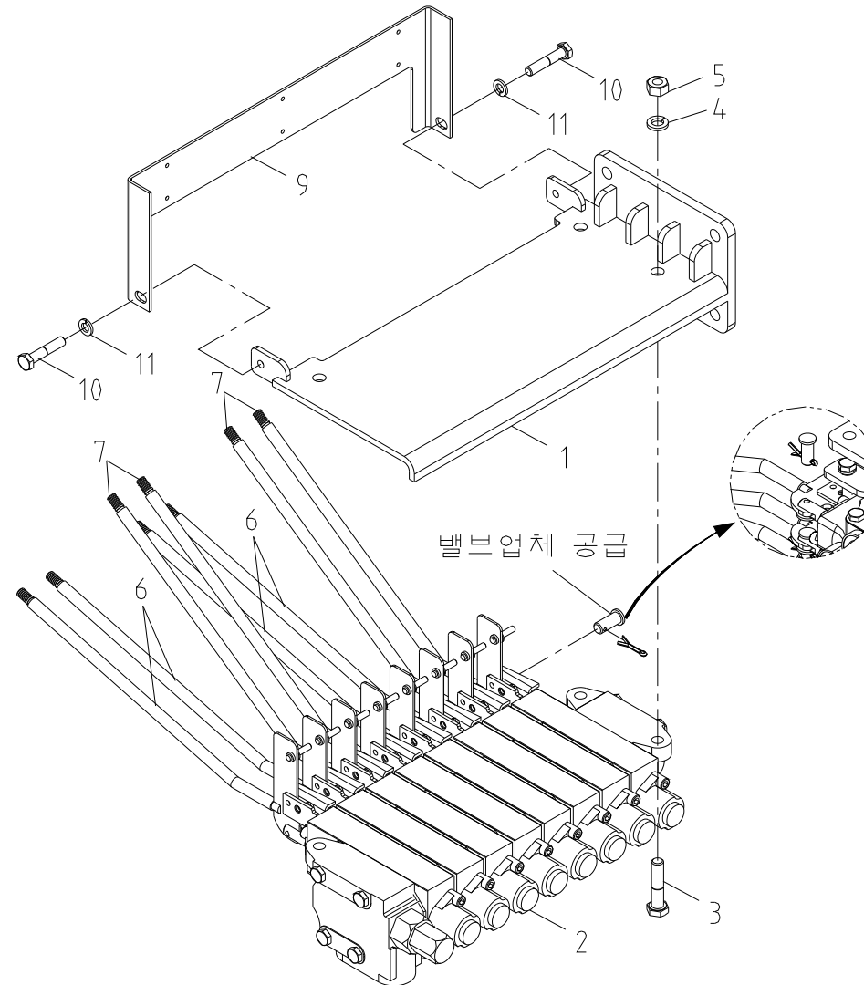
밸브 스텐드 셋 Fig. 3-2-1 SCS1024LSuper VALVE STAND SET
