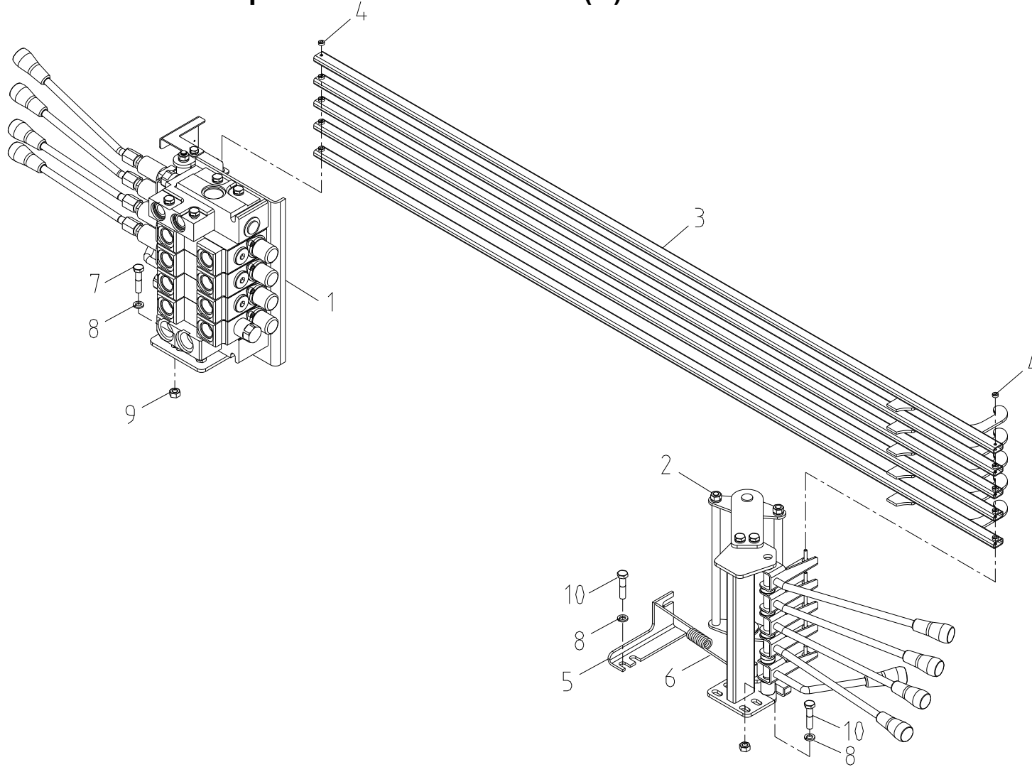
오퍼레이션 조립체 (1) Fig. 3-3 SCS1024LSuper OPERATION ASS'Y (1)
