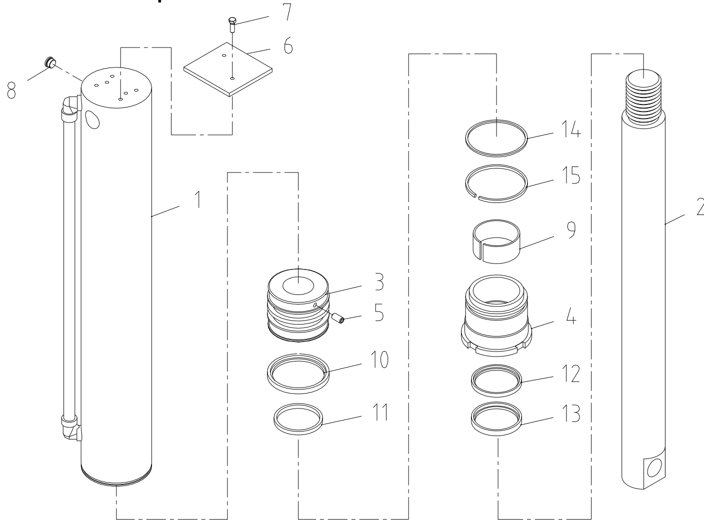
잭 실린더 조립체 Fig. 4-2 SCS1024LSuper JACK CYL' ASS'Y
