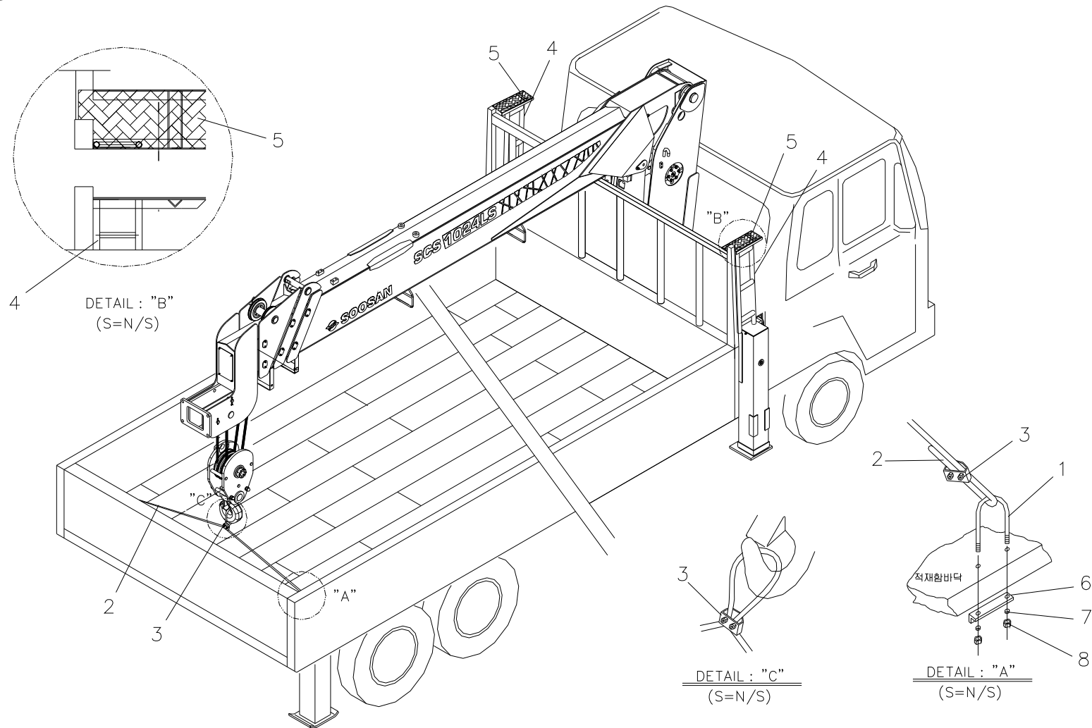
로딩 박스 파트 Fig. 8-5 SCS1024LSuper LOADING BOX PART
