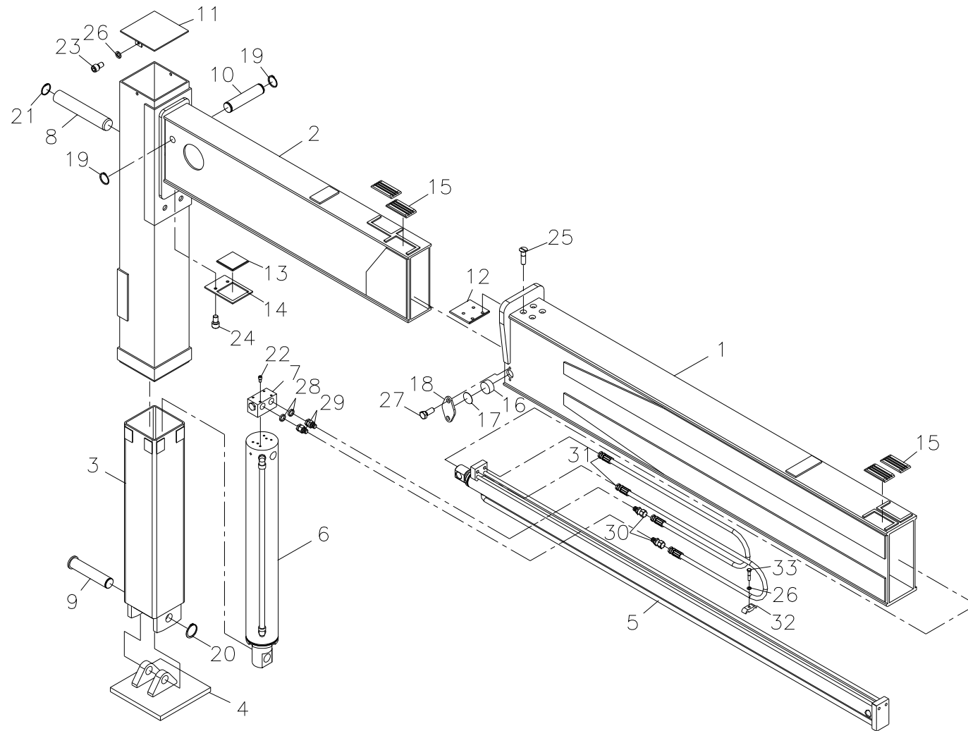
아우트리거 조립체 Fig. 4 SCS1024LSuper OUTRIGGER ASS'Y
