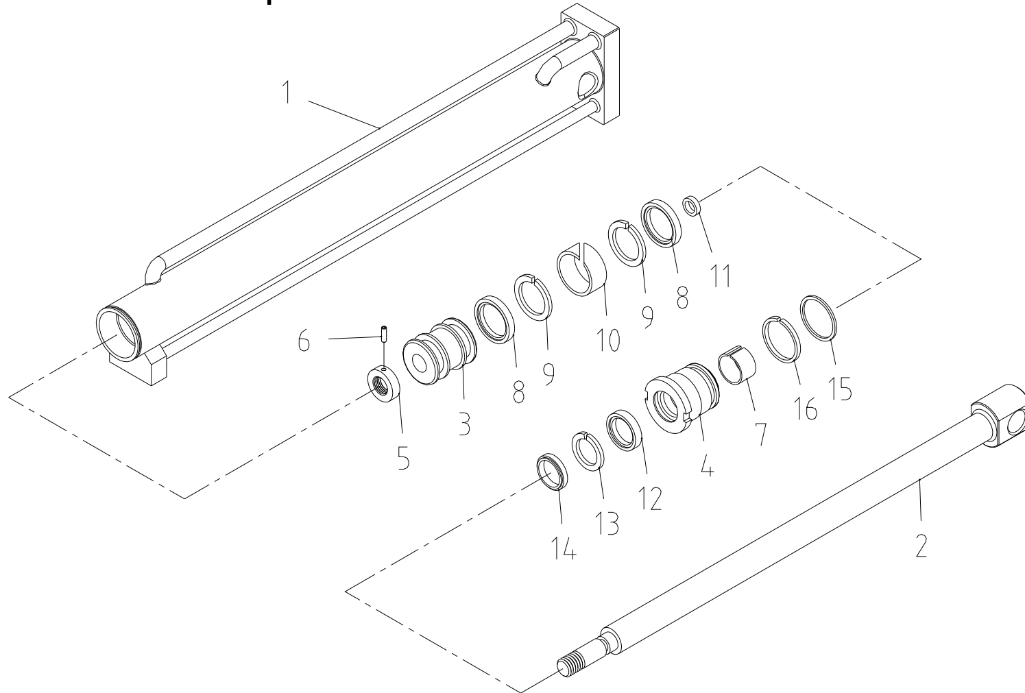
익스펜드 실린더 조립체 Fig. 4-1 SCS1024LSuper EXPAND CYL' ASS'Y
