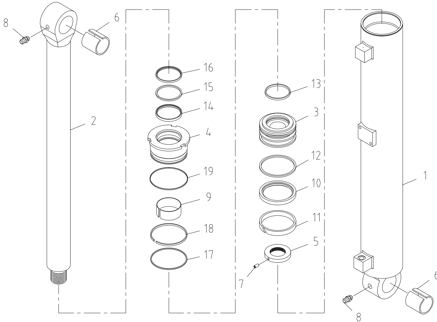
데릭 실린더 조립체 Fig. 2-2 SCS1024LSuper DERRICK CYL' ASS'Y
