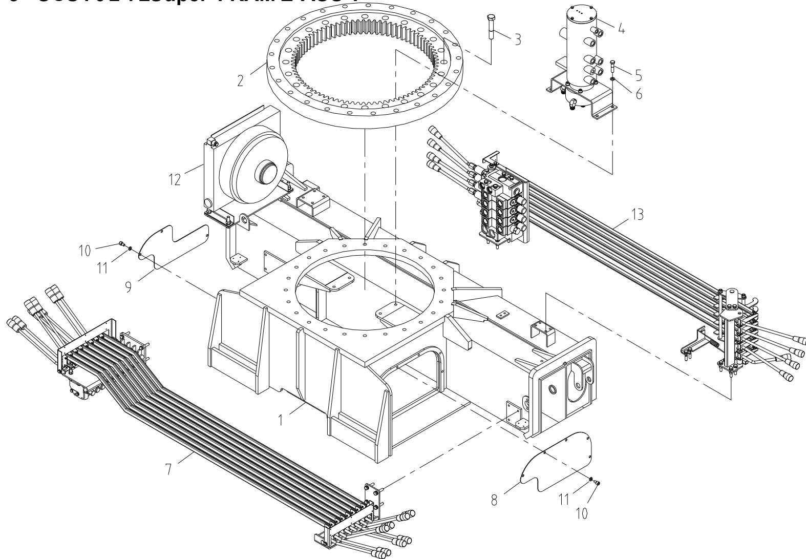
프레임 조립체 Fig. 3 SCS1024LSuper FRAME ASS'Y
